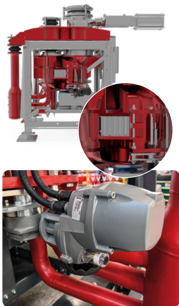
Pfister® AutoGAP 2.1 actuator
